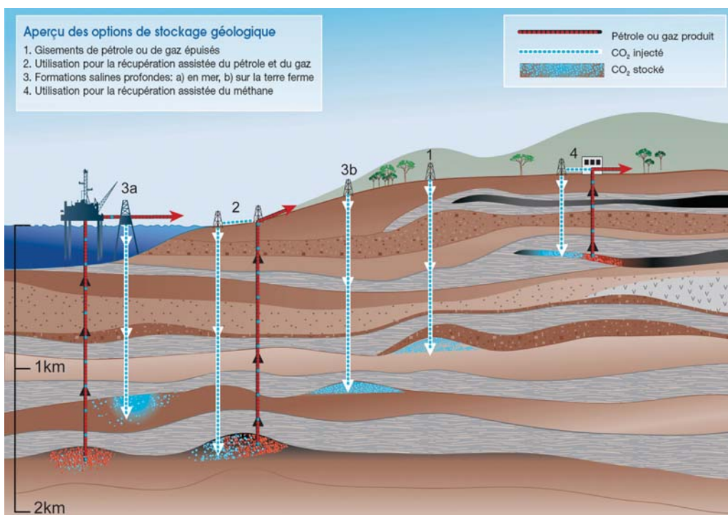
Options de stockage géologique
